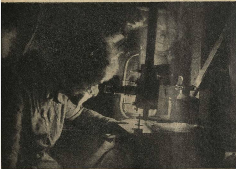
Фототуннелинг
