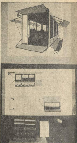
Проект тов. Заонегина. «Стандарт кино и радиопредвижки»
