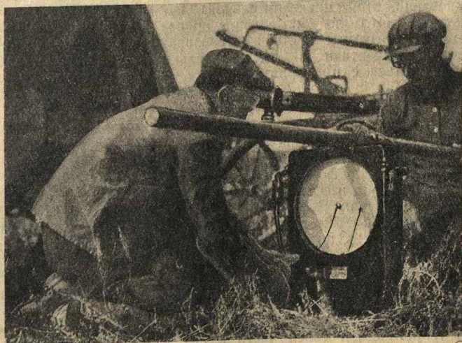
Внизу—испытание силы подъема трактора
