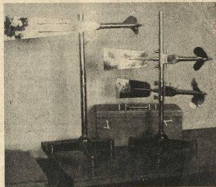
ТСХА. Вертушка для измерения силы движения воды, изготовленная из советских материалов. Фото Нислова
