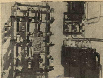
Лаборатория элентротехника
