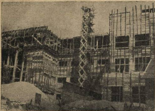
ГЛАВНЫЙ КОРПУС НОВОГО ЗДАНИЯ ГОРНОГО ИНСТИТУТА В СТАЛИНО
