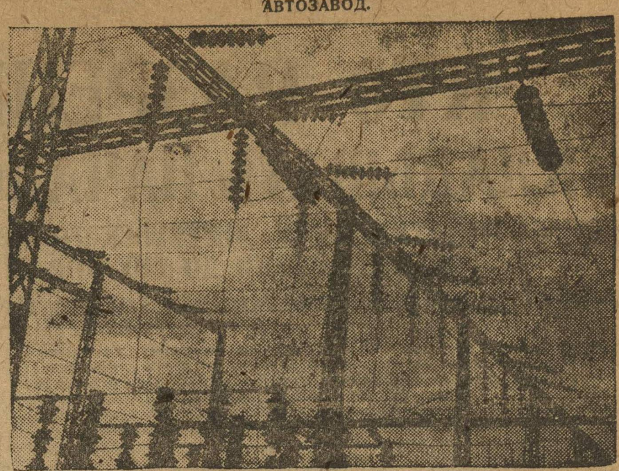
Открытая подстанция автозавода закончена монтажом на три дня раньше срока. Все оборудование подстанции советского производства
