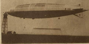
ДИРИЖАБЛЬ ПРИЧАЛИВАЕТ К МАЧТЕ
