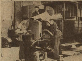
АМО — СБОРКА ГРУЗОВИКА
