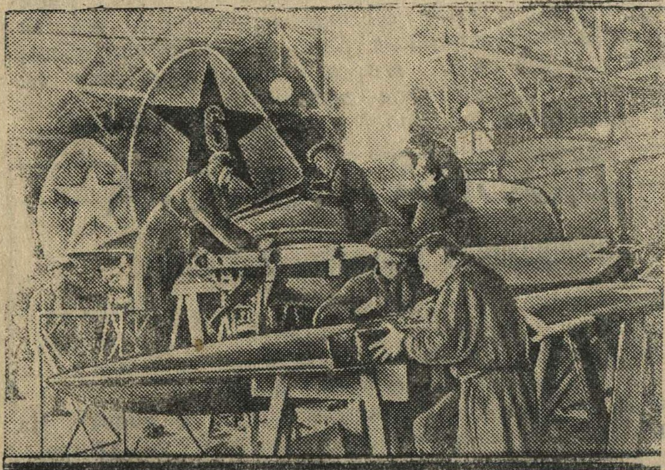
Бригада сборщиков бригадира А. Г. Горохова работающая на сборке истребителей и выполняющая производственные нормы на 250 проц. На переднем плане — бригадир А. Г. Горохов (слева) и сборщик С. Я. Шалдин.
