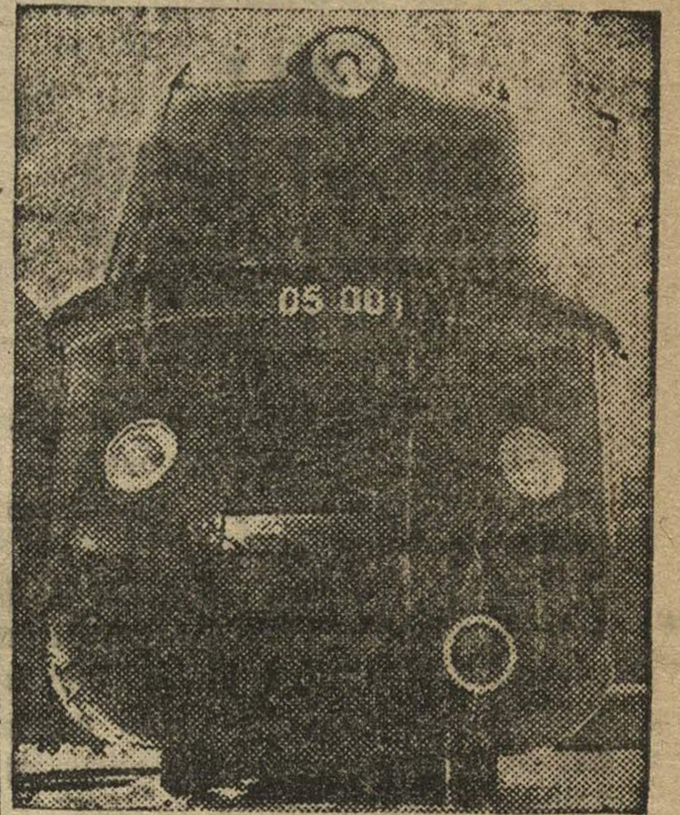
На заводах в Борзиге сконструирован трехосный паровоз обтекаемой формы, показавший на испытаниях предельную скорость в 175 километров в час. Паровоз развивает до 2800 л. с., давление пара составляет 20 кг. на 1 кв. сант. поверхности котла. НА СНИМКЕ: новый паровоз спереди.
