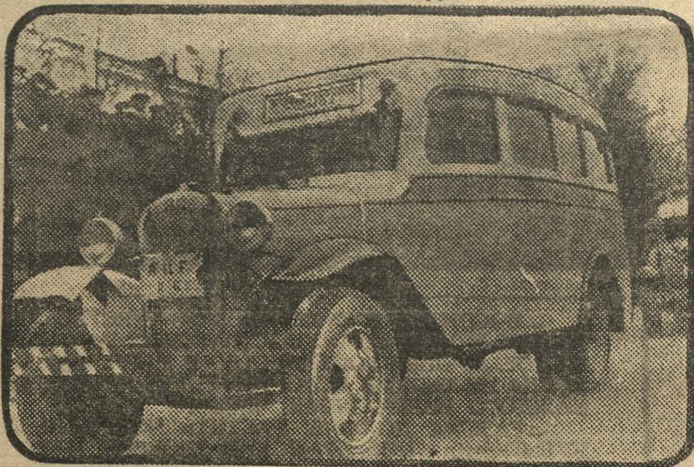
Экспериментальный автобус, модель ГАЗ 12, участвовавший в первомайском параде.
