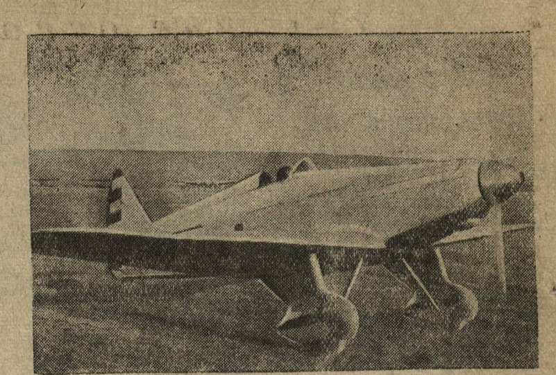
Новый спортивно-тренировочный самолет конструктора А. С. Яковлева. Самолет оборудован автомобильным мотором Горьковского автозавода им. Молотова. Фото А. Межуева. (Фотохроника ТАСС).
