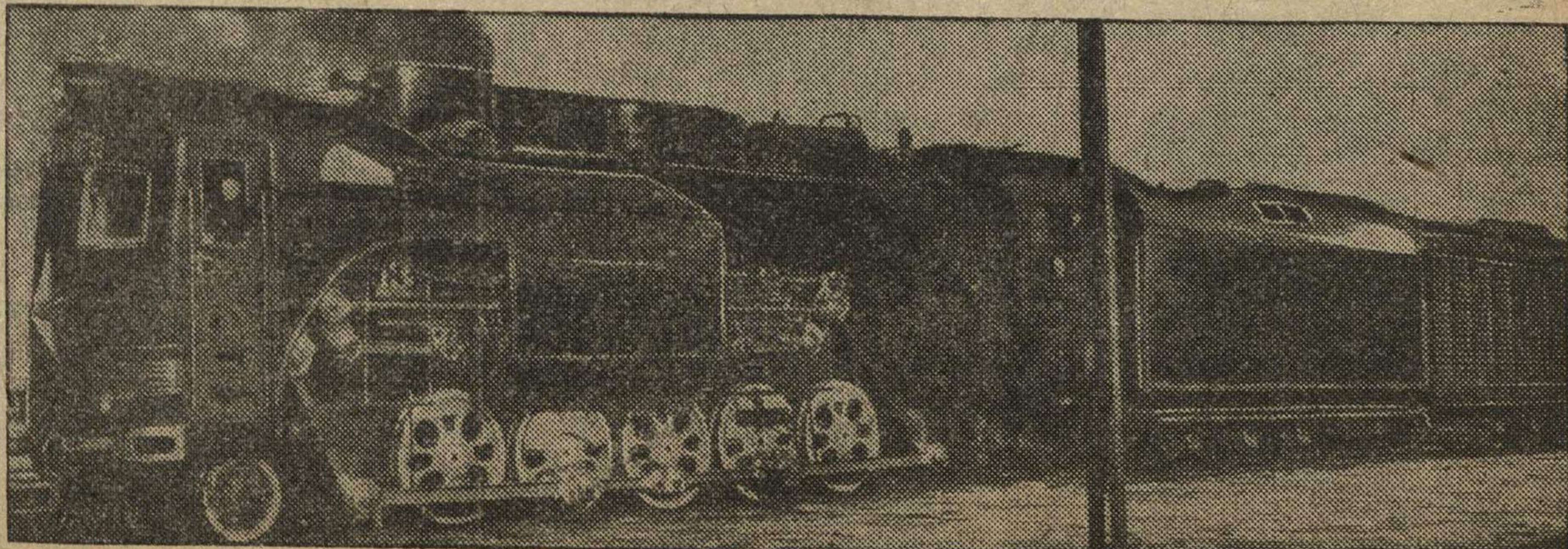
Первый советский товарный тепловоз «Сталинец» с тендерноконденсатором, имеющий комбинированный газопаровой двигатель, работающий на генераторном газе и паре. Этот паровоз построен Коломенским ордена Ленина машиностроительным заводом имени Куйбышева.
