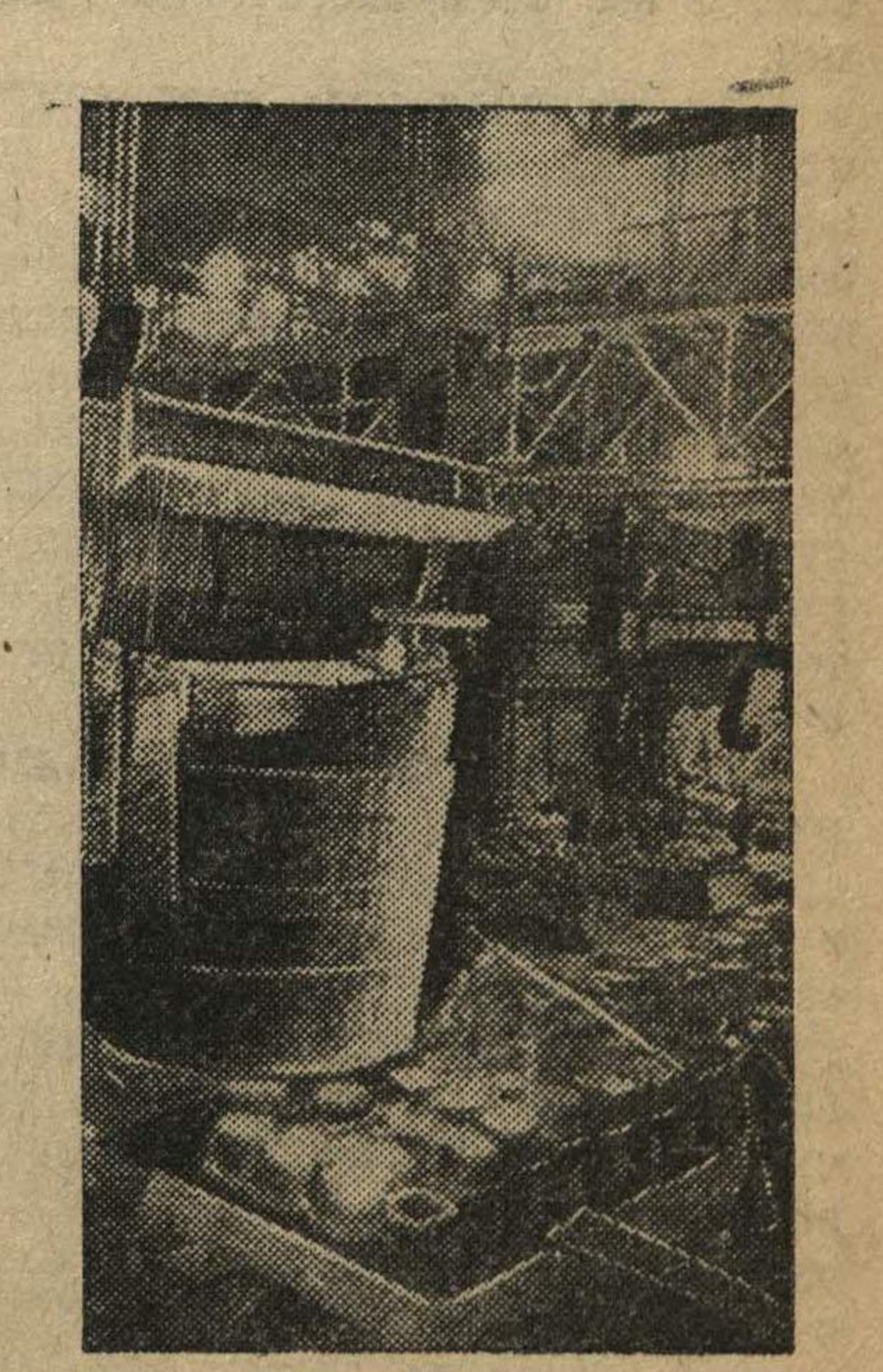
Разливка стали по изложницам в мартеновском цехе № 1 Московского ордена Ленина завода «Серп и Молот».
