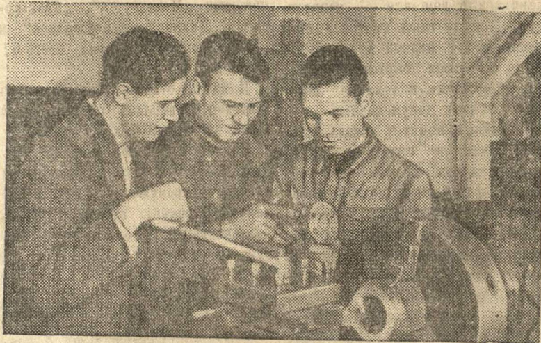
П. С. Безезовский (в центре) знакомит токарей—комсомольцев Л. П. Чудинова и П. М. Махеева со своим приспособленным много-резновой оправкой для токарного станка.
