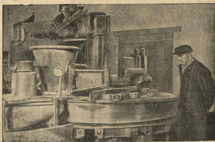
Автоматический брикет-пресс для брикетирования чугушной стружки, установленный в копровом цехе Челябинского тракторного завода имени Сталина. Перелавка в вагранках чугушной стружки даст заводу около 100 тыс. рублей экономии в год.
