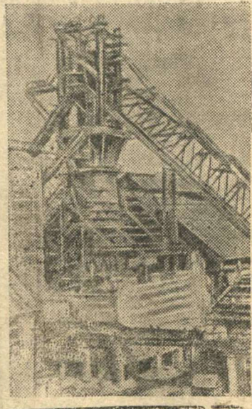
Строительство второй доменной печи Челябинского металлургического завода.
