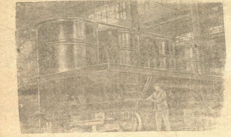
Мощный углеазгрузочный четырехбукерный вагон для Горловского коксохимического завода, построенный коллективом котельного цеха Красноярского машиностроительного завода сверх плана. Фото С. Малобичко. Фотохроника ТАСС
