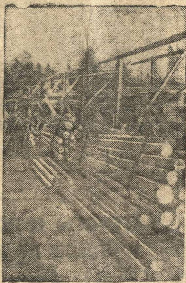
Погрузка леса на поезд подвешиваемой дороги.
