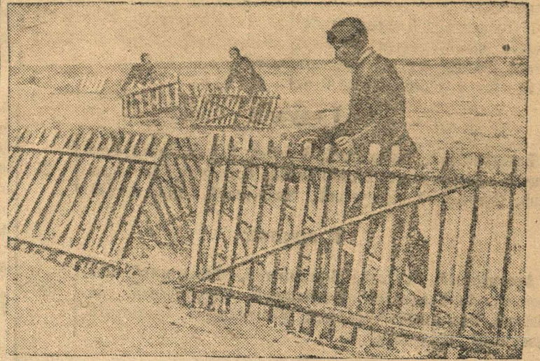
Расстановка щитов для снегозадержания. Фото А. Маклецова.
