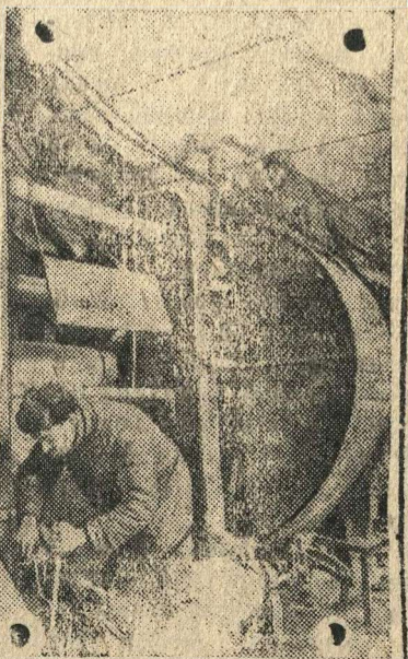
Монтируются машины и агрегаты в восстанавливаемом цехе ситценабивной фабрики «Пролетарка».
