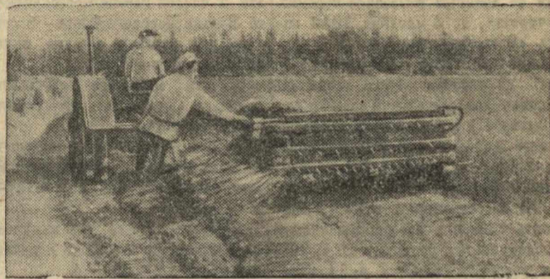
Уборка льна льчотеребилкой в колхозе «Совет», Сернурского района, Марийской АССР.
