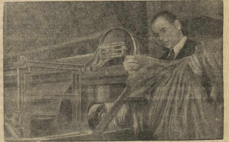
Тов. П. К. Кондрашук осматривает льноволокно, обработанное на льнотрепальной машине «ЛТМ» его конструкции. (Фото-Клише ТАСС).
