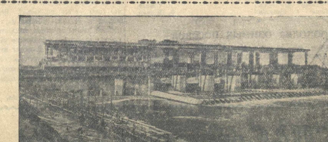
Общий вид строительства ГЭС Угличского гидроузла и железобетонной плотины № 1. Фотокашине ТАСС.
