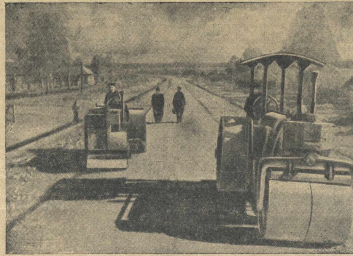
На строительстве дороги Горький—Муром—Кулебаки. Уютна готового участка дороги в Вачском районе. Фото М. Опец.
