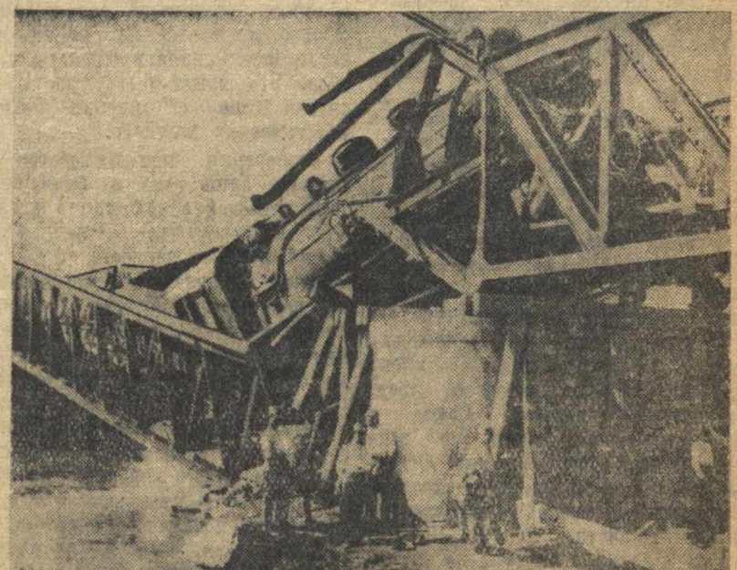
Железнодорожный мост на линии Бейпин-Ханькоу, разрушенный китайской авиацией с целью воспрепятствовать продвижению японских войск.
