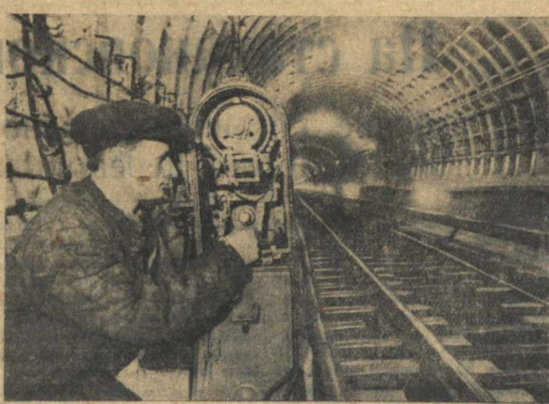
Строительство Московского метро второй очереди. На снимке: начальник автоблокировки Покровского участка тов. К. В. Телешов проверяет установку «Автоостоп» и сигнализацию. Союзфото.
