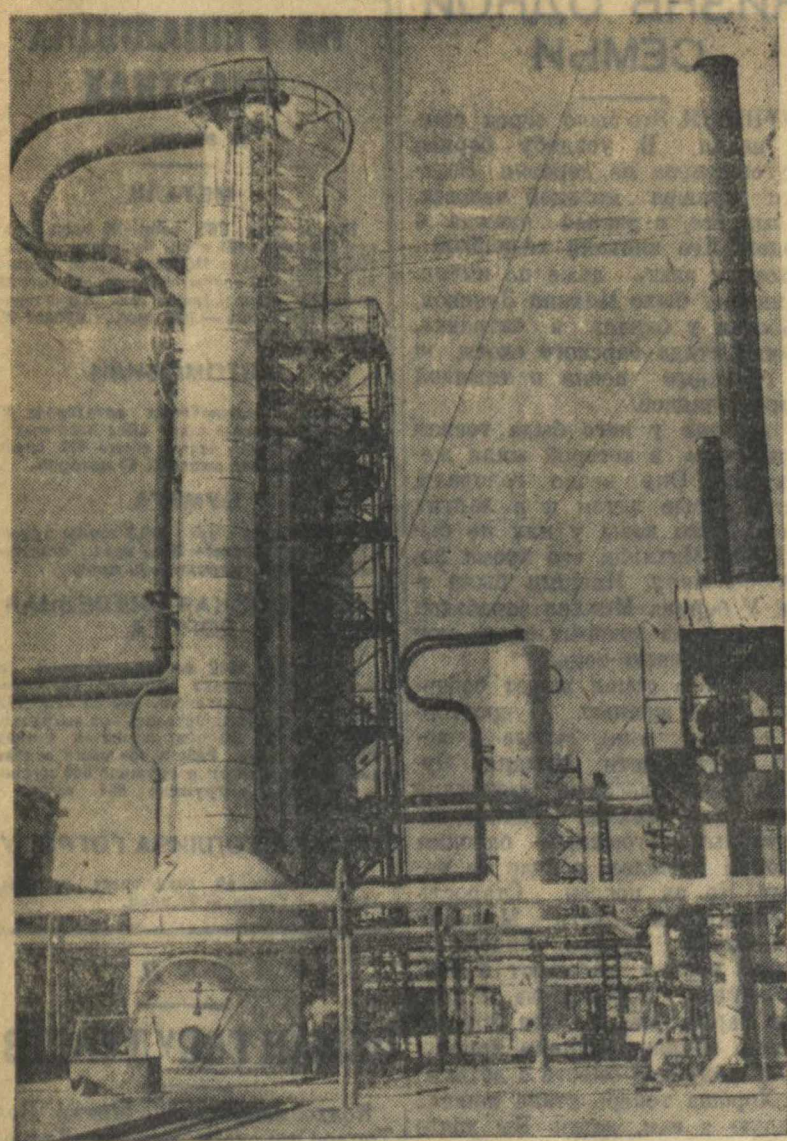
К пятилетию доклада товарища Сталина: «Итоги первой пятилетки». Отечественный кренинг-установка для переработки нефтепродуктов на кренинг-заводе им. Вавилова (Баву).
