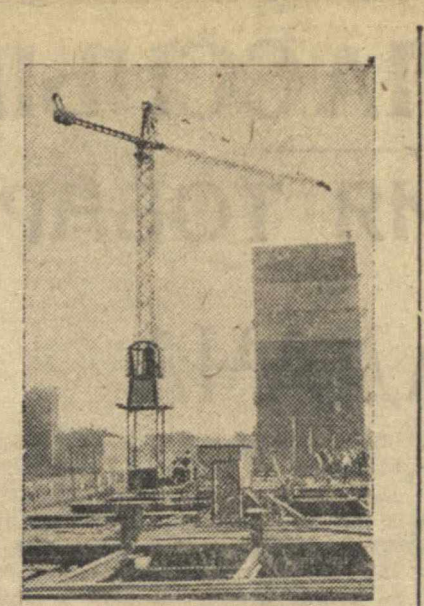
Московский машиностроительный завод «Красный металлист» выпускает первый башенный кран, поднимающий до трех тонн груза на высоту 40 метров и обслуживающий рабочие участки в радиусе 20 метров. На снимке: первый башенный кран завода «Красный металлист» на строительном доме по 1-й Мещанской ул. в Москве.
