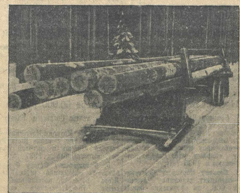
Одна из лесовозных машин, работающая на вывозке леса с участка (Уваровский механизированный участок Кузбасского лескомбината). Фото А. Капелюша.
