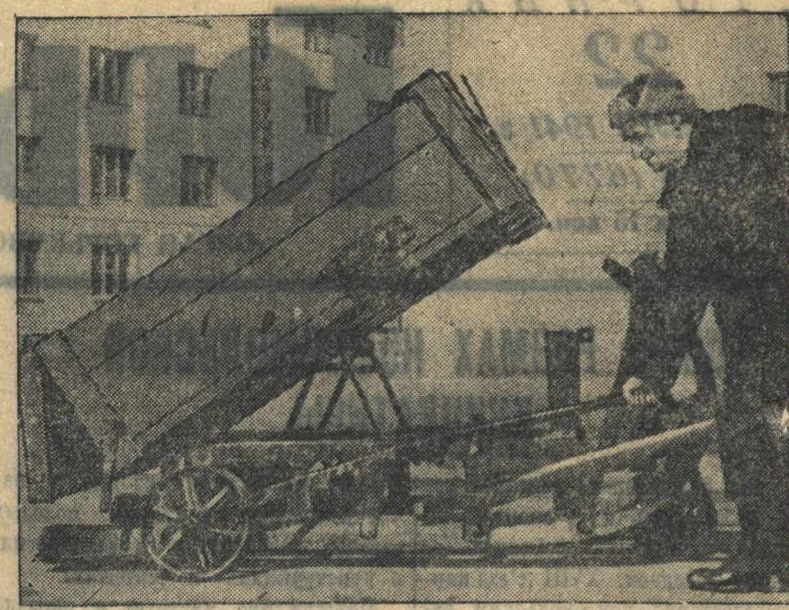
Работник Стройгаза И. С. Прозоров сконструировал удобные для подвозки строительных материалов сани, которые при помощи особого рычага — переключателя можно при необходимости превратить в тележку. На снимке: И. С. Прозоров у своего изобретения. Фото В. Храмова.
