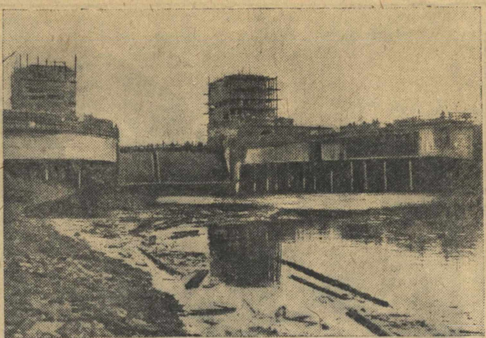
На канале Москва—Волга. Первые волжские воды подходят к головному шлюзу канала (№ 1). Фото Ф. Кислова (Союзфото).
