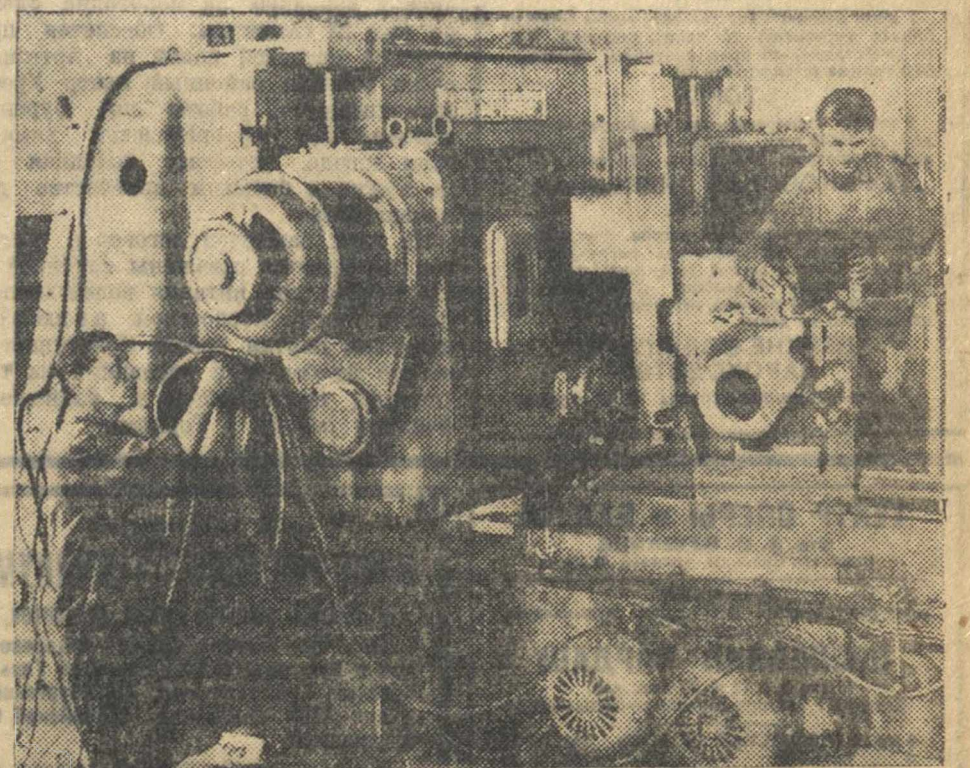
Сейчас на станкозаводе идет монтаж нового станка типа 6С—52. Станок изготавливается для Харьковского тракторного завода. На снимке: монтаж станка, бригадир монтажа М. Л. Логинов (слева) и ученик слесаря А. П. Соколкин (справа). Фото А. Капелюша.
