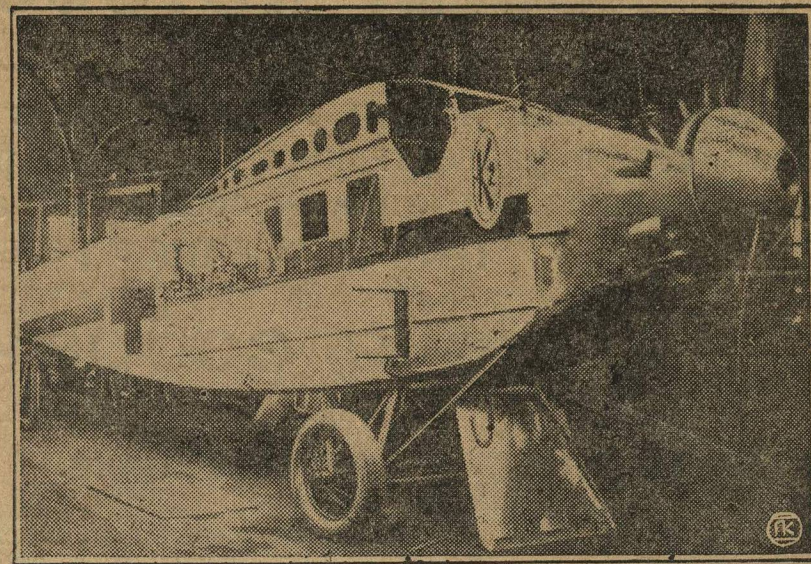
В Харькове недавно построен первый советский санитарный самолет по плану конструктора тов. Калинина. На снимке — самолет после выпуска.
