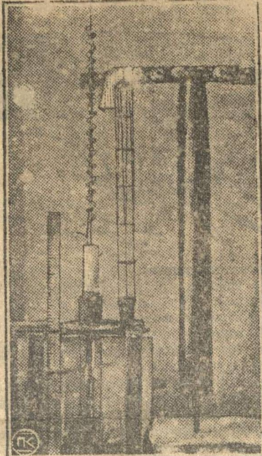
Детали 100 киллов. лампы («Ильич»), сконструированной Бонч-Бруевичем. Слева нить канала, лдущая спирально вокруг кварцев. стержня. Посредине сетка лампы, справа — анод, служащий и внешней оболочкой лампы.
