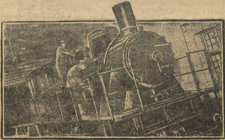
ЗАВОД ИМ. ЛЕНИНА — один из ленинградских машино-строительных заводов, точно выполняет промфинплан. На снимке: ударники за сборкой очередного вновь выпускаемого паровоза.
