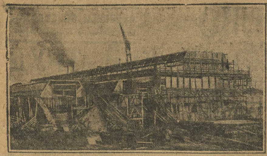
СОВЕТСКАЯ СТРАНА ИНДУСТРИАЛИЗИРУЕТСЯ. В Москве находится в разгаре строительства будущий гигант — автосборочный завод. НА СНИМ-КЕ: постройка главных механических корпусов.
