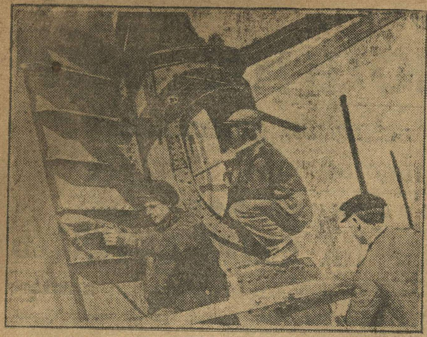
НА ПОСТРОЙКЕ МОСТА ЧЕРЕЗ ОКУ. На снимке: установка аппарата для опускания кессонов.
