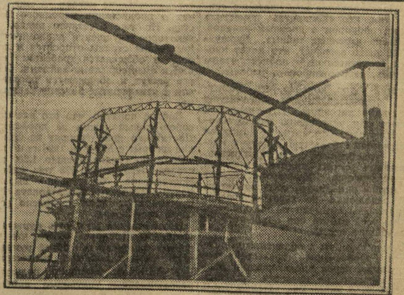
Газохранилище, строящееся на заводе «им. Октябрьской Революции».
