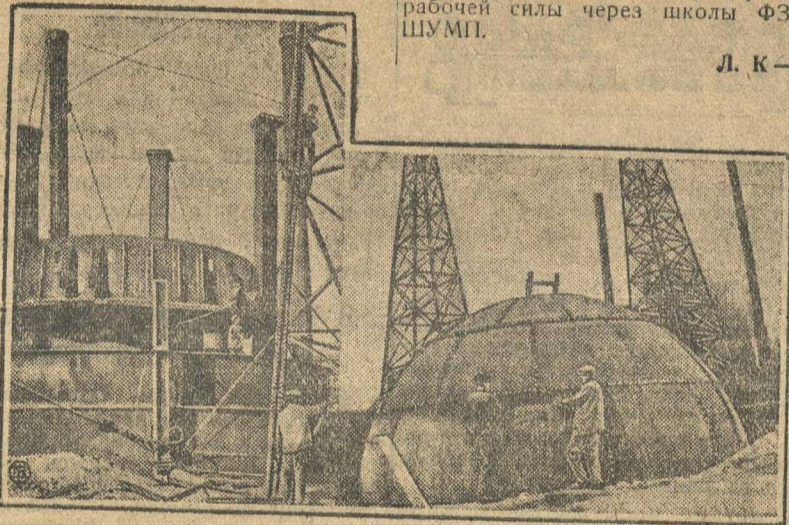
КРУПНОЕ СТРОИТЕЛЬСТВО В МЕТАЛЛУРГИИ. На Макеевском заводе им. Томского (Донбасс) широко развернулись работы по постройке новой мощной доменной печи № 5. На снимке: слева — фундамент и средняя часть корпуса домны № 5, справа — клепка крышек «кауперов».
