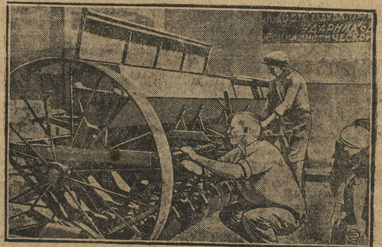
КОМСОМОЛЬЦЫ СЕЛЬМАШСТРОЯ XVI ПАРТСЪЕЗДУ. Ударная бригада комсомольцев Сельмашстроя (Ростов н/Дону) досрочно выпустила первую советскую тракторную сеялку. Сеялка выпущена, как подарок XVI съезду партии.
