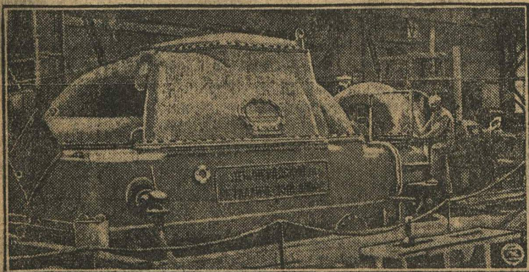
ПОДАРОК К XVI ПАРТС'ЕЗДУ ОТ ЗАВОДА ИМ. СТАЛИНА. Завод им. Сталина в Ленинграде закончил постройку 2-й турбины в 24.000 киловатт. Турбина собрана на 1 мес. раньше срока. НА СНИМКЕ: турбина на стенде во время испытания.
