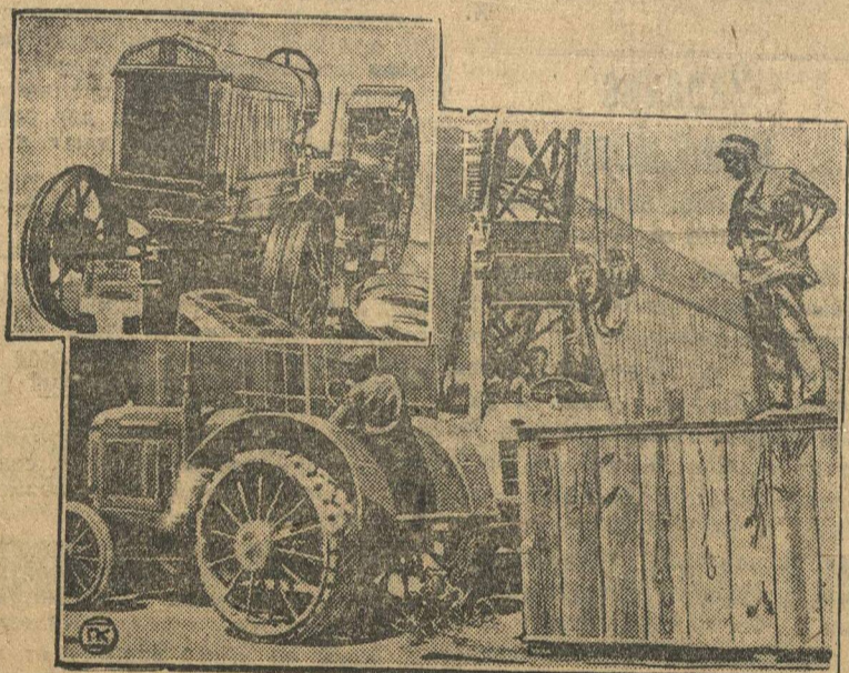
В связи с предстоящим 15 июня пуском Сталинградского тракторного завода им. Дзержинского всем цехам даны производственные задания. В первый же месяц работы, т. е. по 15 июля, завод должен выпустить 100 тракторов. На снимке: разгрузка оборудования для Тракторостроя, вверху в углу—1-й опытный трактор, выпущенный Тракторостроем.
