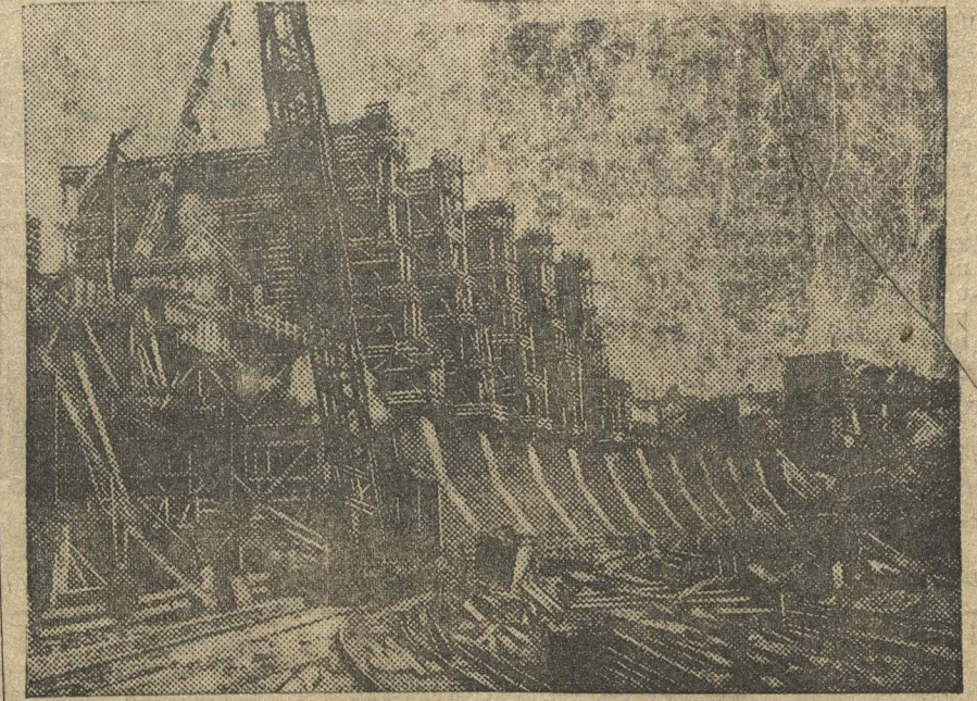
НА ДНЕПРОСТРОЕ. Бетонировка бычков плотины левого берега.
