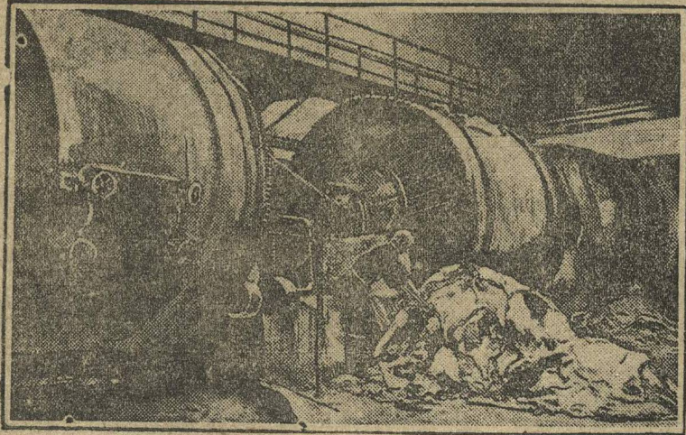
НАШИ ДОСТИЖЕНИЯ. ТАГАНРОГ. ТЕХНИЧЕСКИЙ ДИРЕКТОР ТАГАНРОГСКОГО КОЖЕВЕННОГО ЗАВОДА ТОВ. ВАЙЗБЕРГ ИЗОБРЕЛ ТАК НАЗЫВ. «ЗОЛЬНЫЙ БАРАБАН» ДЛЯ ДУБЛЕНИЯ КОЖИ. ИЗОБРЕТЕНИЕ ПОЗВОЛИЛО СОКРАТИТЬ ПРОЦЕСС ДУБЛЕНИЯ КОЖИ С 10 СУТОК ДО 16 ЧАСОВ. НА СНИМКЕ: ИЗОБРЕТЕНИЕ ТОВ. ВАЙЗБЕРГА — «ЗОЛЬНЫЕ БАРАБАНЫ».
