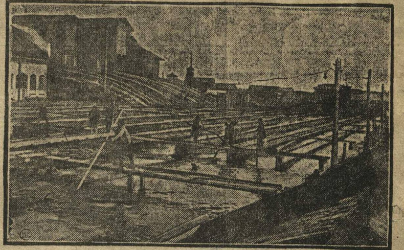
МЕХАНИЗАЦИЯ ЛЕСОПРОМЫШЛЕННОСТИ СССР. На лесозаводе № 25 Северолеса в Архангельске построен первый в Сев. крае верхне-наливной отопленный бассейн. Бассейн на 2 метра выше уровня реки. Подача бревен в бассейн производится элеваторами. На снимке: верхне-наливной отопленный бассейн. Слева—лесозавод.
