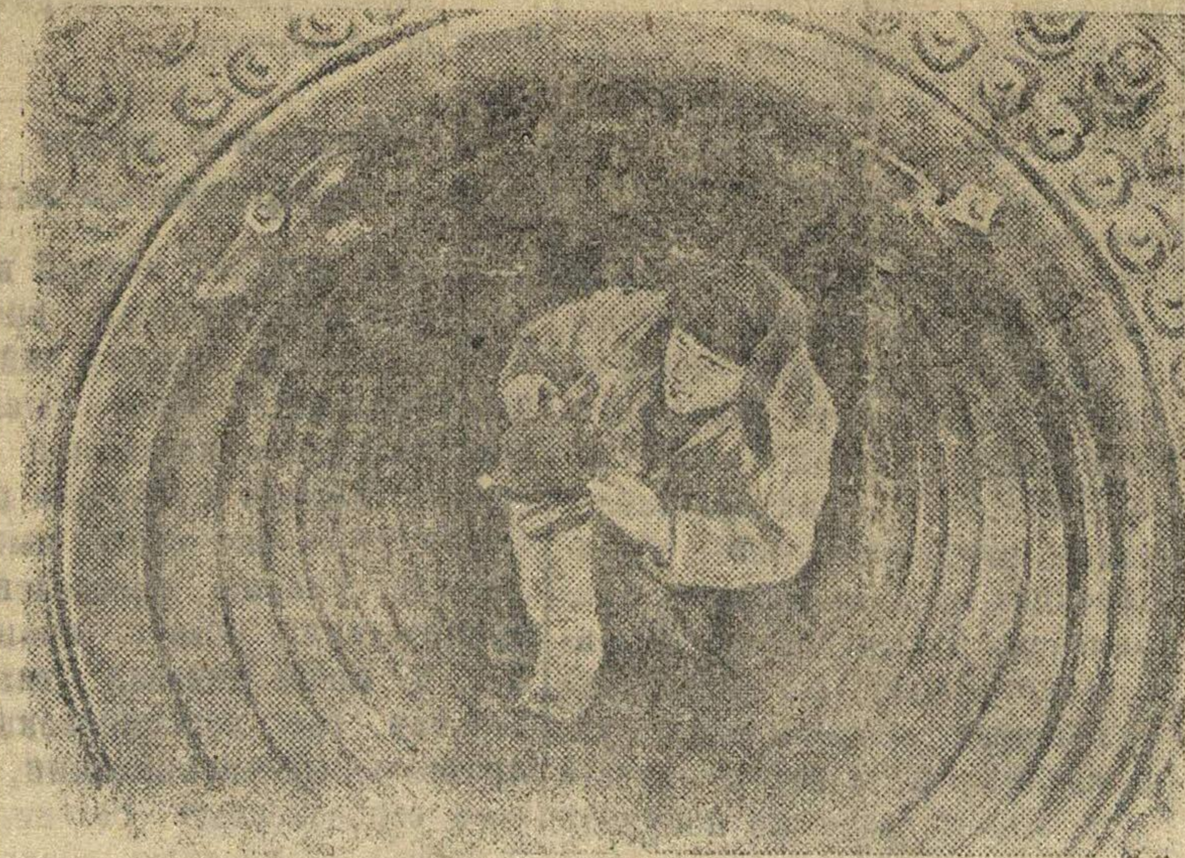
На снимке: Студент энергетического факультета И. Ф. Кольдин за восстановлением котла парового двигателя. Фото Н. Фигуркина. Фотохроника ТАСС
