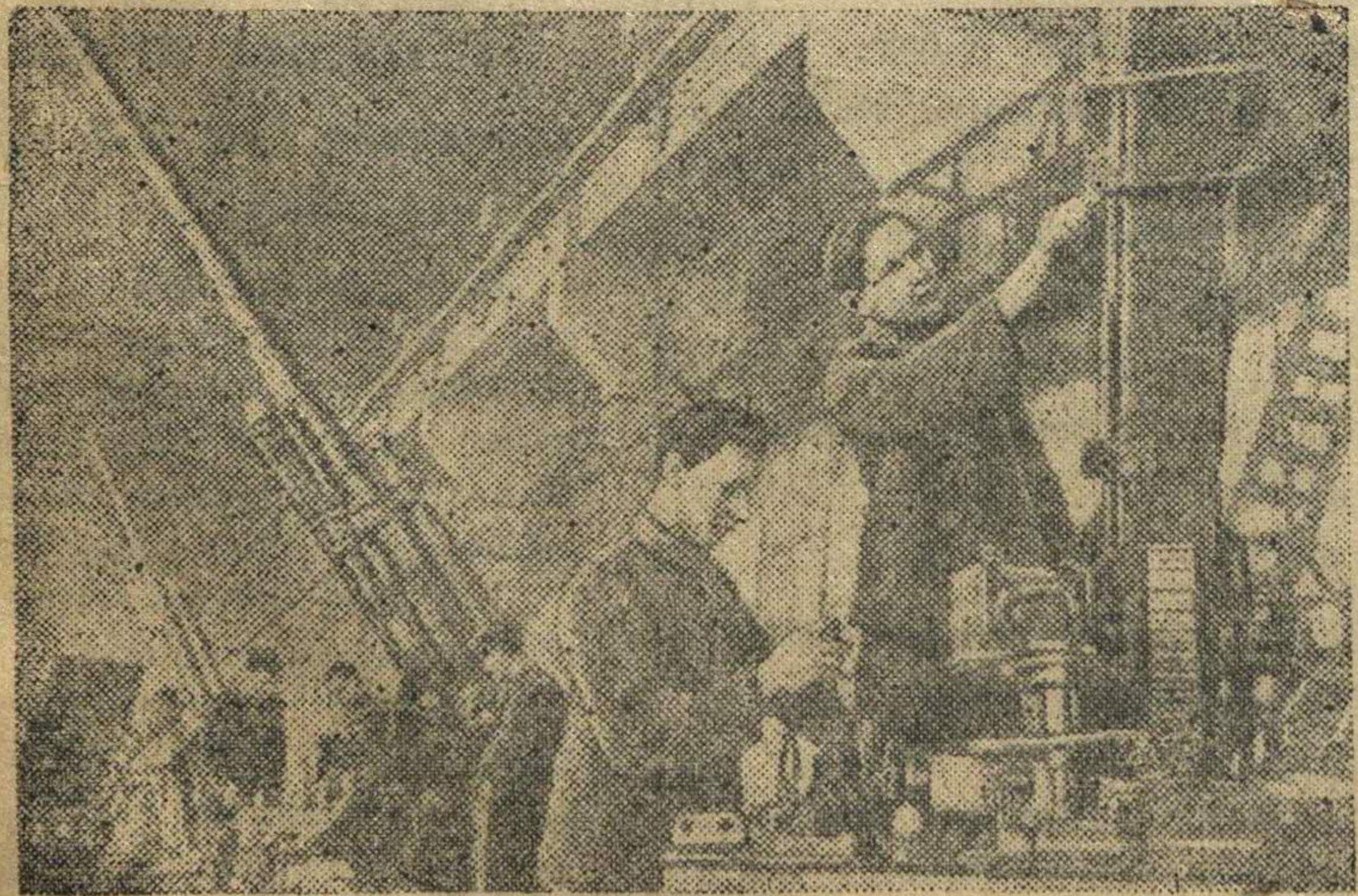
Нский артиллерийский завод. Сборка зенитных орудий. На переднем плане слесари-сборщики стахановцы Б.А. Сибирков (слева) и комсомолец К. В. Кондривов.
