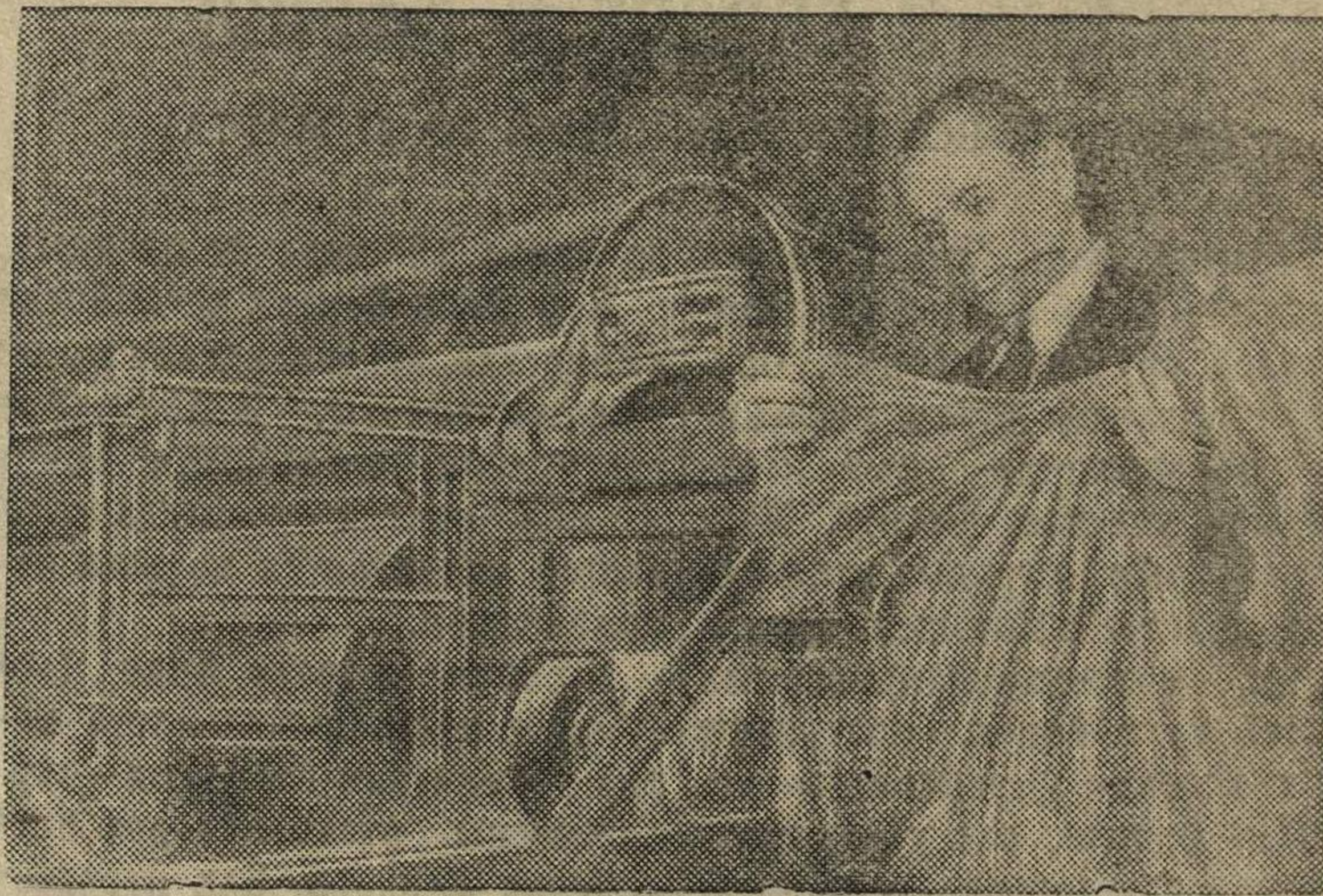
На снимке: Тов. П. К. Кондрашук осматривает льноволокно, обработанное на льнотрепальной машине «ЛТМ» его конструкции. Фото Н. Чамова. Фото ТАСС.
