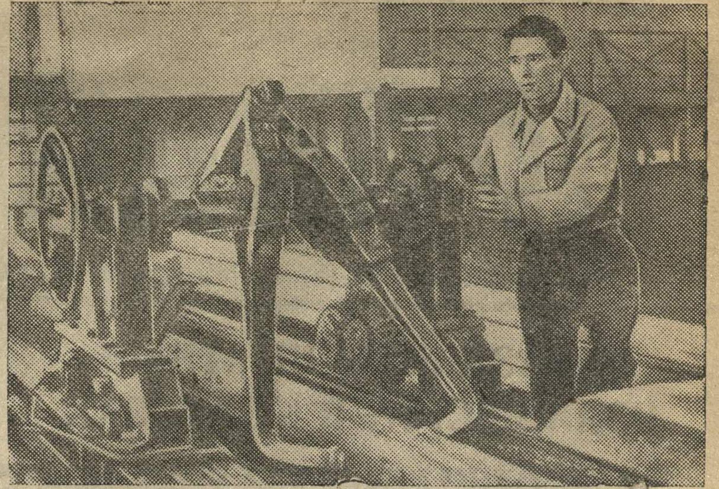
НА СНИМКЕ: техник-рационализатор лесопильного завода имени Куйбышева (Сталинград) тов. А. М. Егоров, сконструировавший портативную комлеву тележку для подачи бревен к лесопильной раме. Годовая экономия от одной тележки составляет 26 тысяч рублей.
